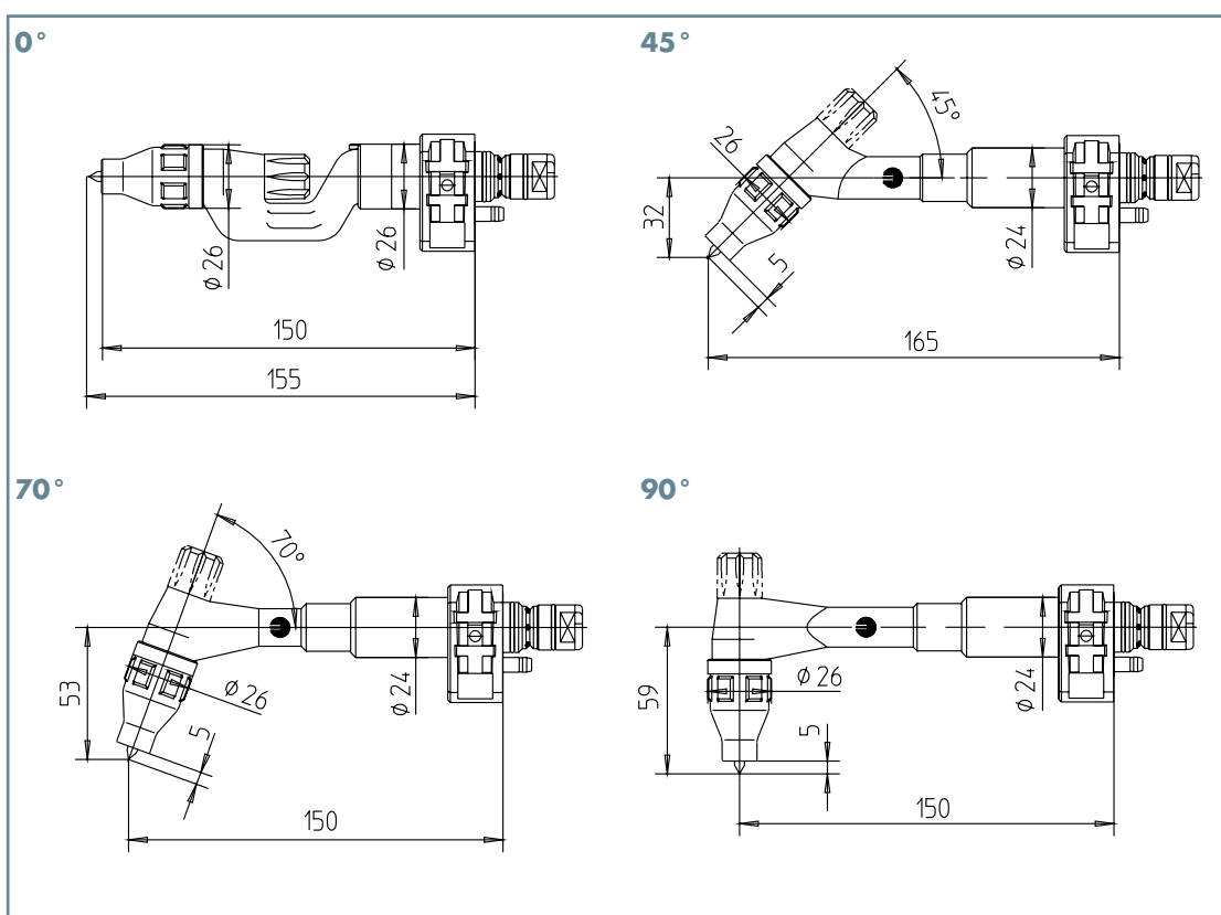
Maßskizze ABITIG® WH 400 W
