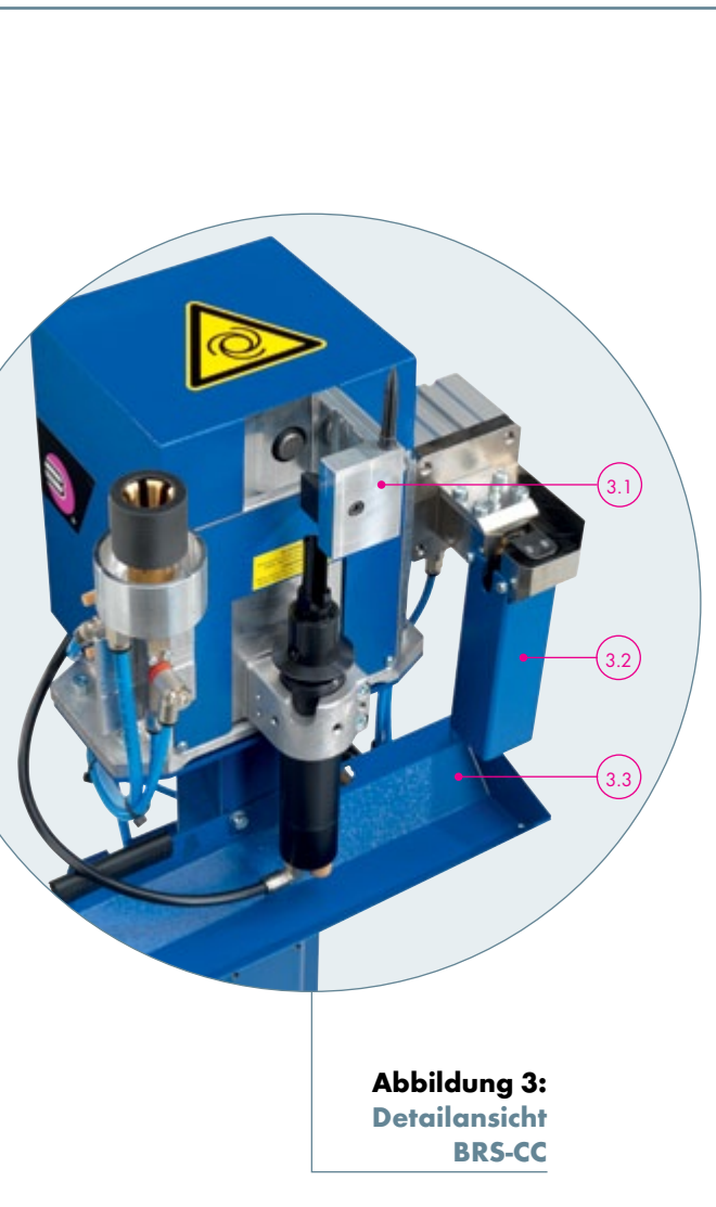
Abbildung 3: Detailansicht BRS-CC
