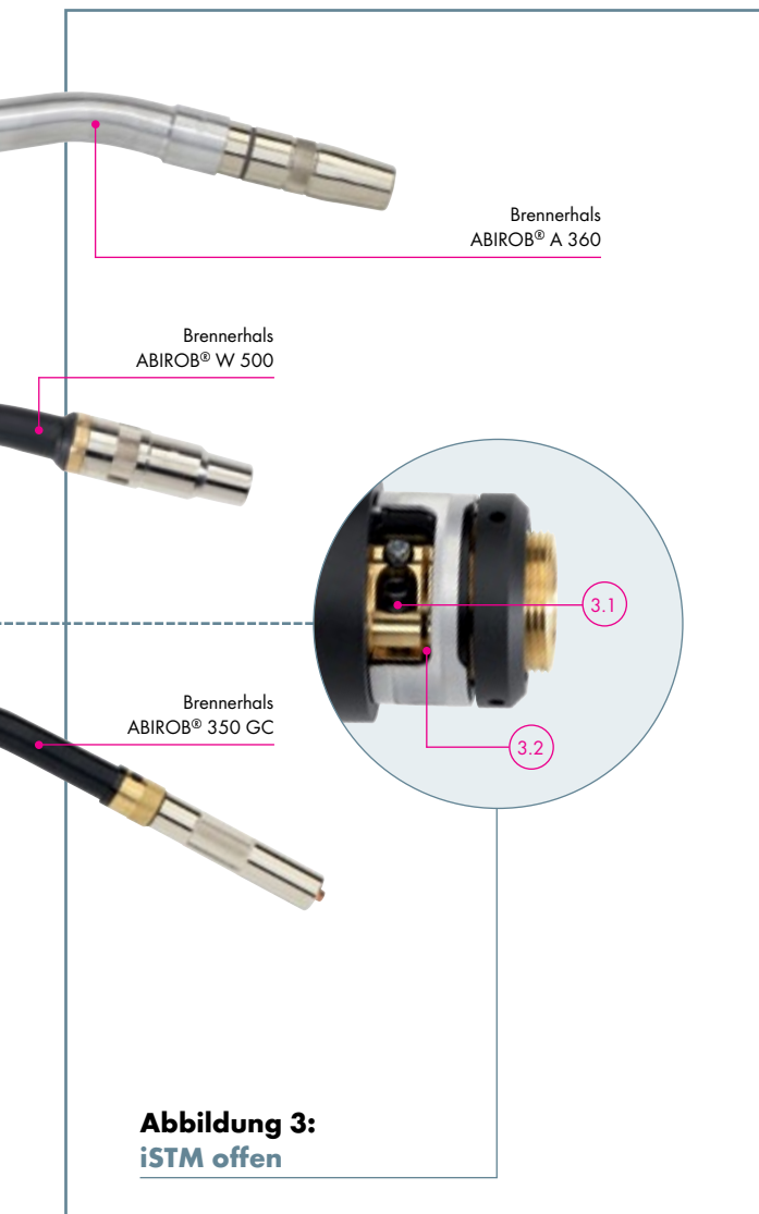
Abbildung 3: iSTM offen
