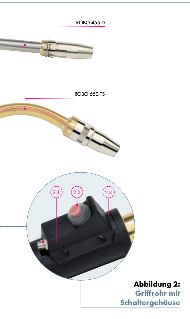
Abbildung 2: Griffrohr mit Schalergehäuse
