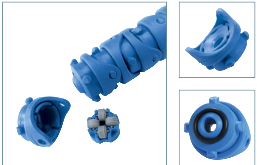
Abbildung 3: Anschluss G 1/8" konvex (Einzelteile)
